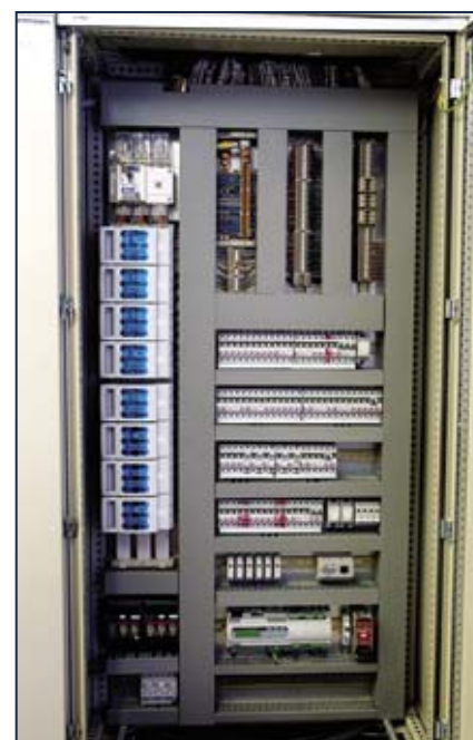
Primer stikalnega bloka razsvetljave s krmilnim sistemom
